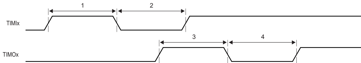
图 11-51. Timer Timing
