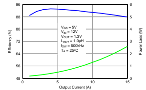
典型电源块效率与功率损耗
