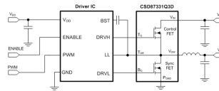
典型电路
