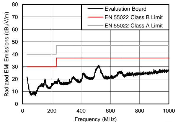
辐射发射图
