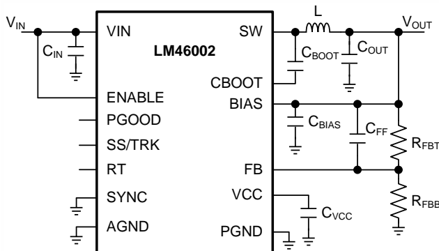
简化原理图
