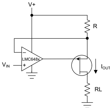
图 7-21. 范围广泛的合规电流源
