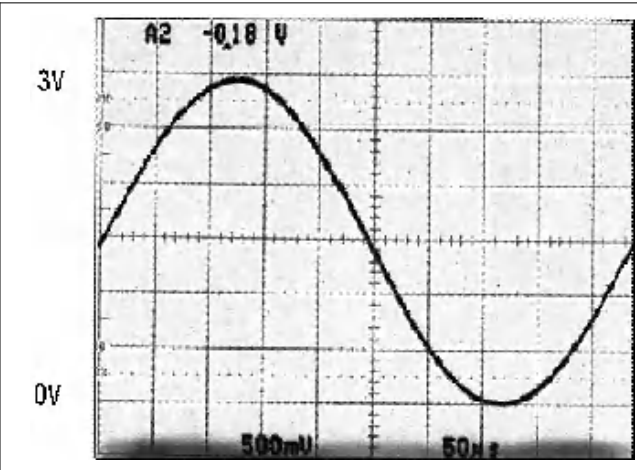
图 7-16. 轨到轨输出
