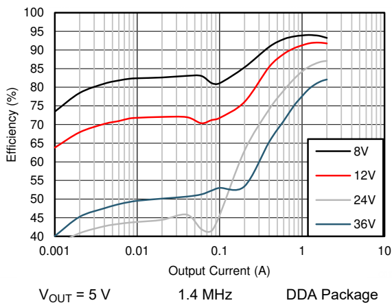
图 9-9. Efficiency
