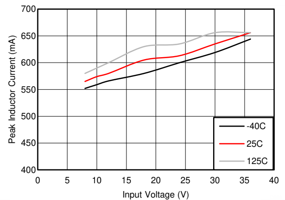
图 7-6. I_{PEAK-MIN}
