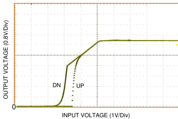
图 7-5. UVLO Thresholds
