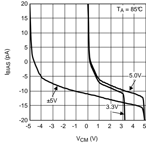
图 8. 输入偏置电流与 V_{CM} 间的关系
