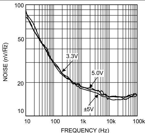
图 30. 输入电压噪声与频率间的关系
