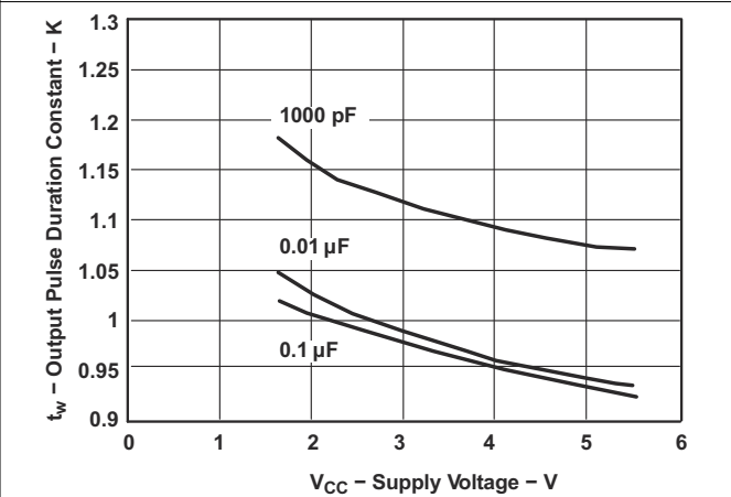
图 5-6. 输出脉冲持续时间常数与电源电压的关系
