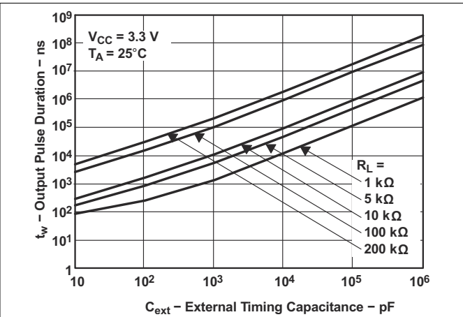
图 5-4. 输出脉冲持续时间与外部时序电容的关系
