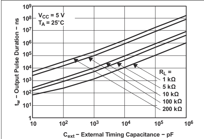
图 5-5. 输出脉冲持续时间与外部时序电容的关系
