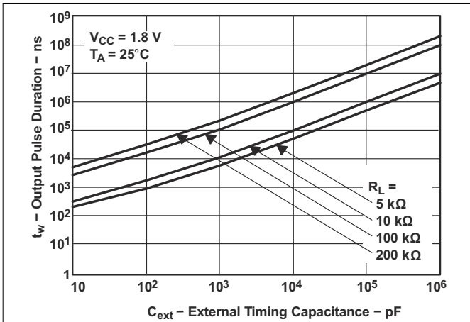
图 5-3. 输出脉冲持续时间与外部时序电容的关系
