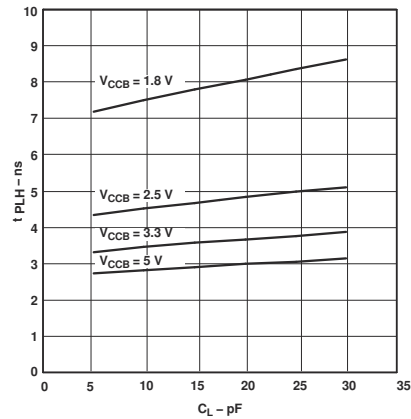
图 5-6. 低电平到高水平 (A 到 B) 的典型传播延迟与负载电容间的关系 T_A = 25^\circ\text{C} 、 V_{CCA} = 2.5\text{V}
