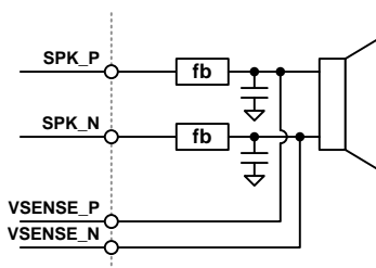
图 31. V-Sense Connections
