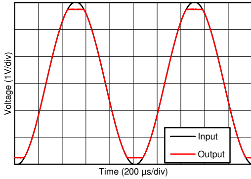
图 5-25. 无相位反转
