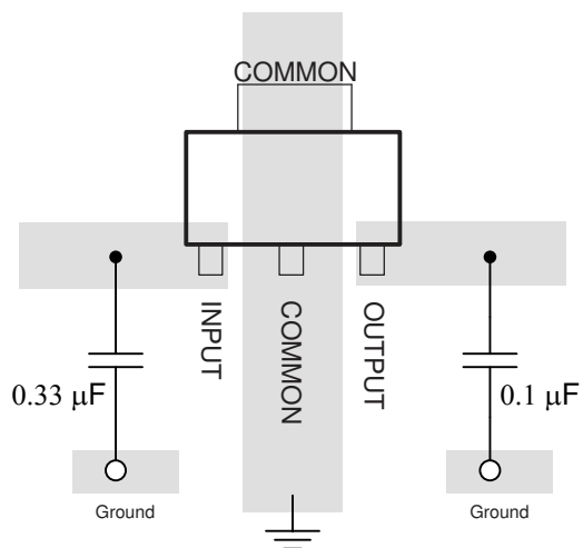
图 7-12. Layout Diagram
