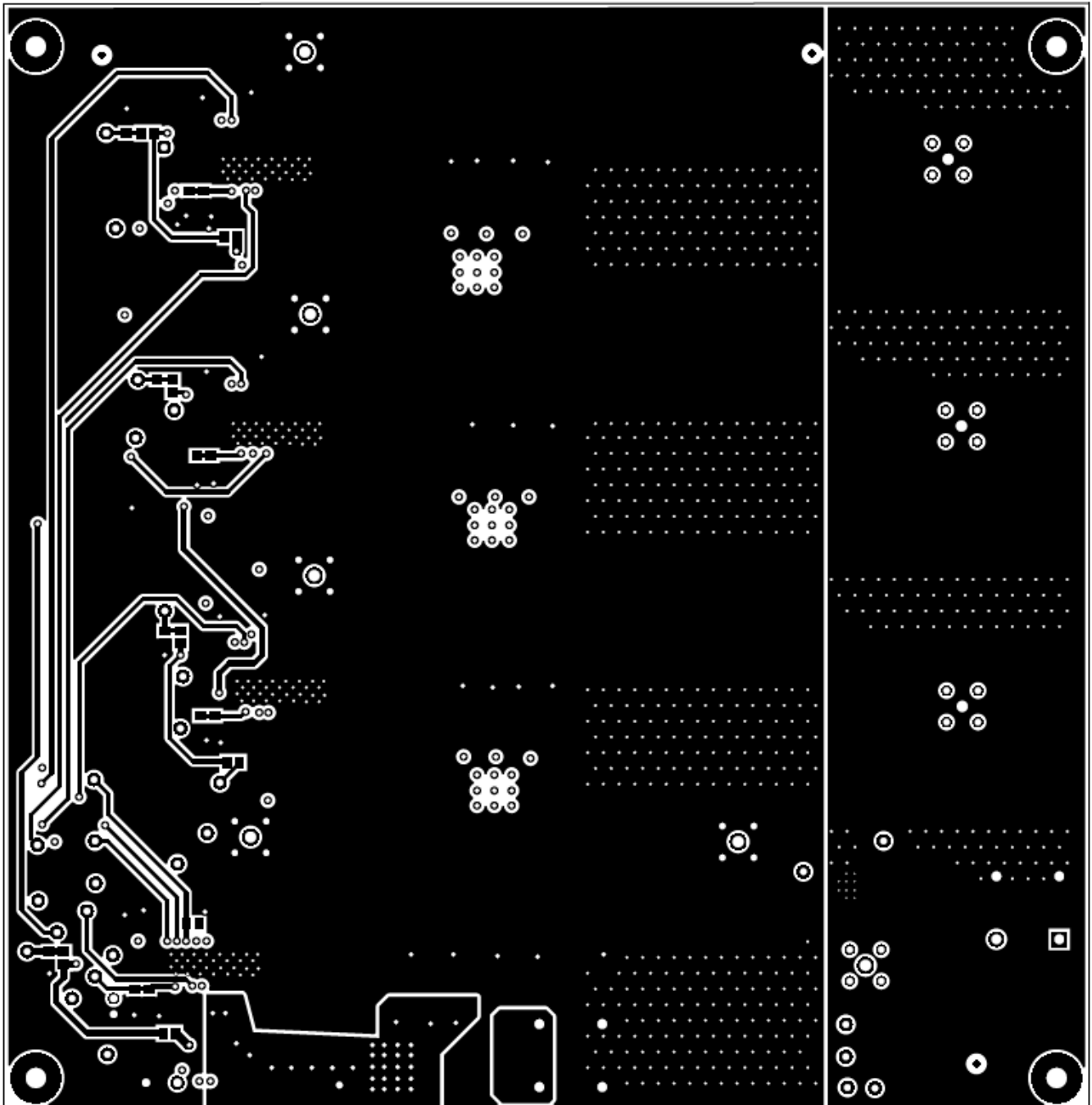
Figure 24. Bottom Layer
