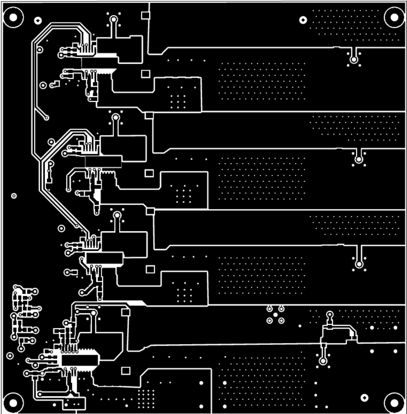
Figure 17. Top Layer
