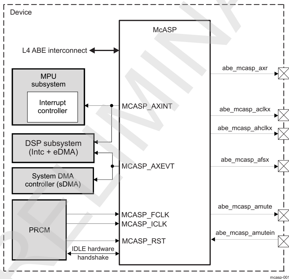
Figure 23-185. McASP Module
