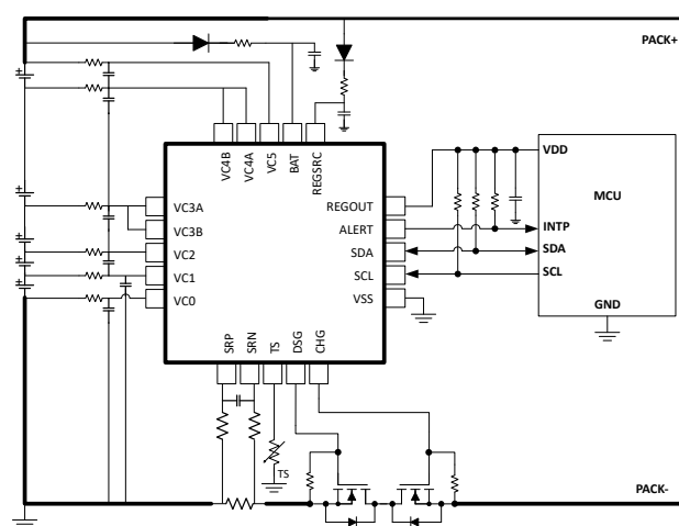
图 3-1. 简化原理图
