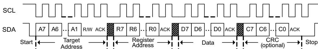
图 7-2. I 2 C 写入
