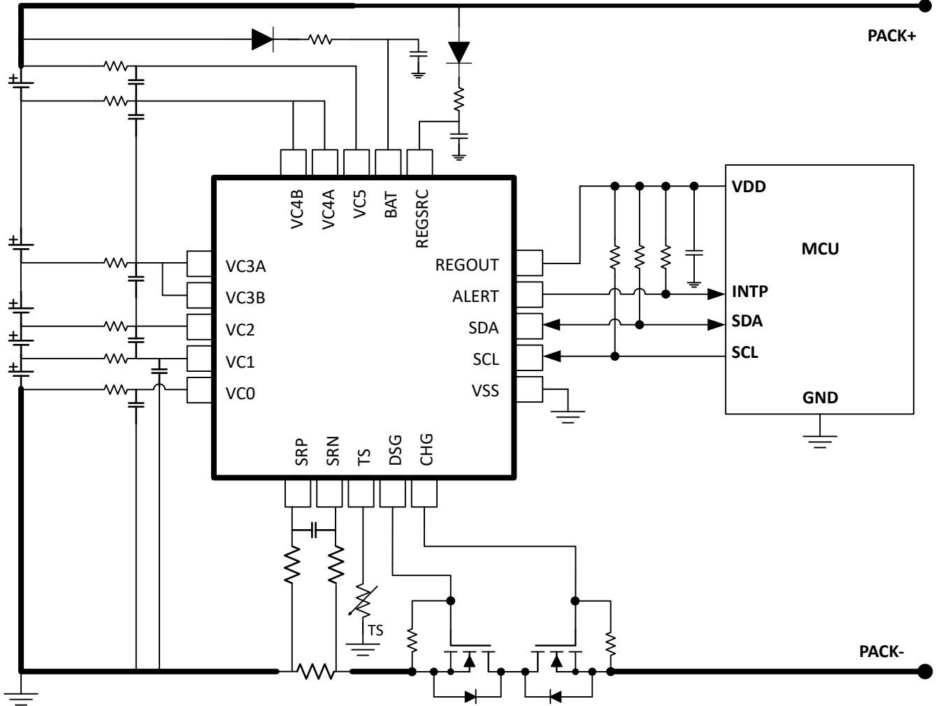
图 8-1. BQ76905 5 节串联电芯典型实现方式 (简化原理图)
