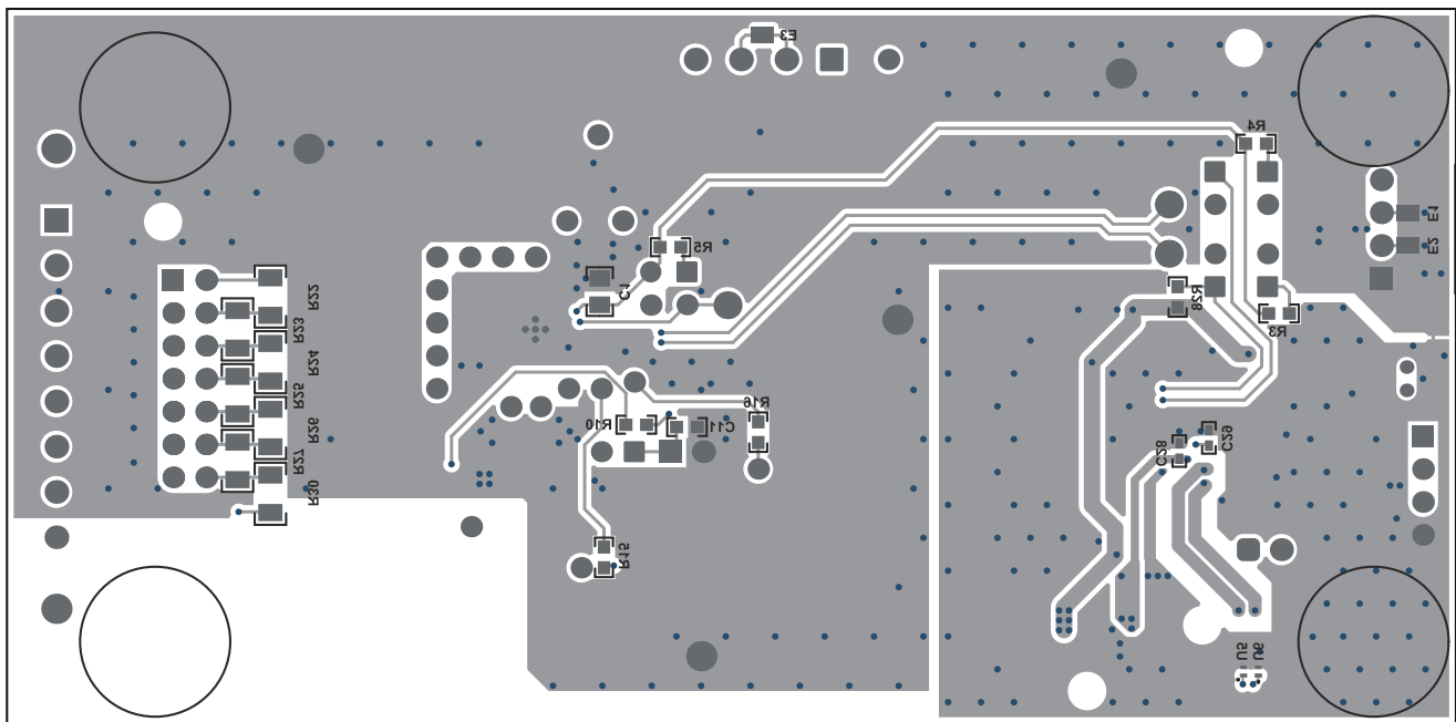
图 8-10. BQ76905 两层电路板布局布线 - 底层
