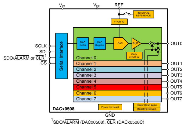
简化方框图
