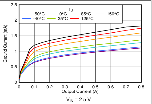
图 7-8. I_{GND} vs I_{OUT}
