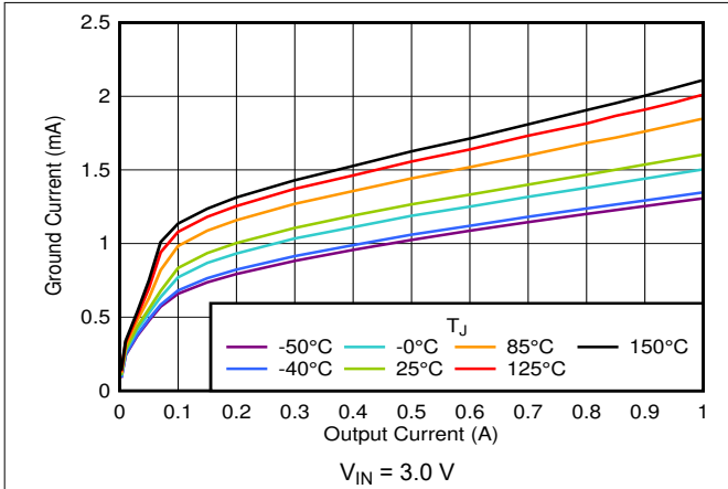
图 7-7. I_{GND} vs I_{OUT}
