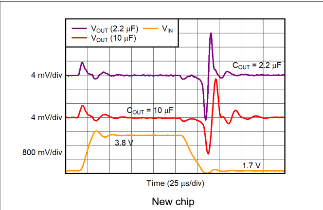
图 5-38. V_{IN} Line Transient
