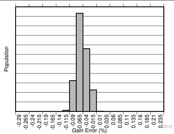
图 6-14. 增益误差产生分布图 A4
