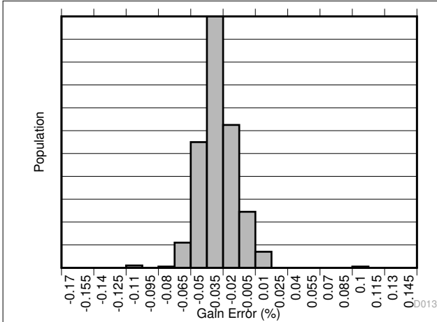
图 6-13. 增益误差产生分布图 A3
