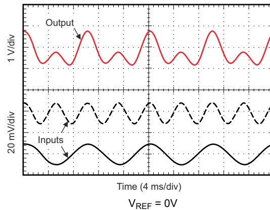
图 8-4. 电流求和应用输出响应 (A2 器件)
