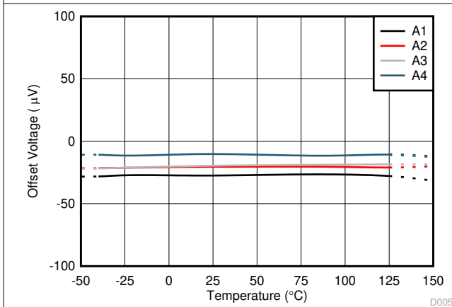
图 6-5. 失调电压与温度间的关系
