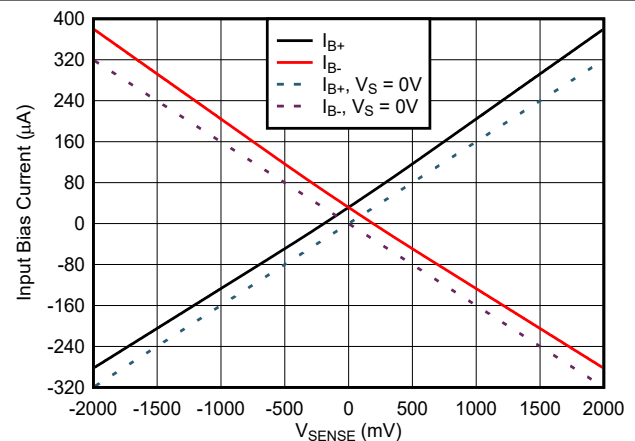
图 7-18. INA296x1 输入偏置电流与 V_SENSE 间的关系
