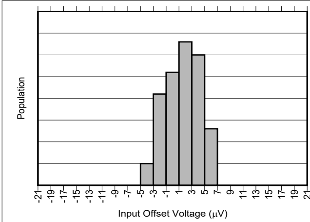
图 7-1. INA296A1 输入失调电压产生分布图
