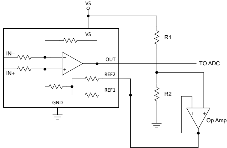
图 8-8. 使用电阻分压器和运算放大器缓冲器来设置基准
