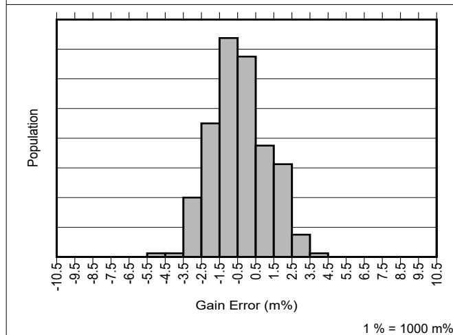
图 7-11. INA296A4 和 INA296A5 增益误差产生分布图
