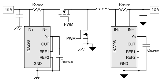
典型应用 - 直流/直流转换器
