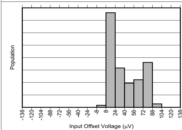
图 7-3. INA296A3 和 INA296A4 输入失调电压产生分布图
