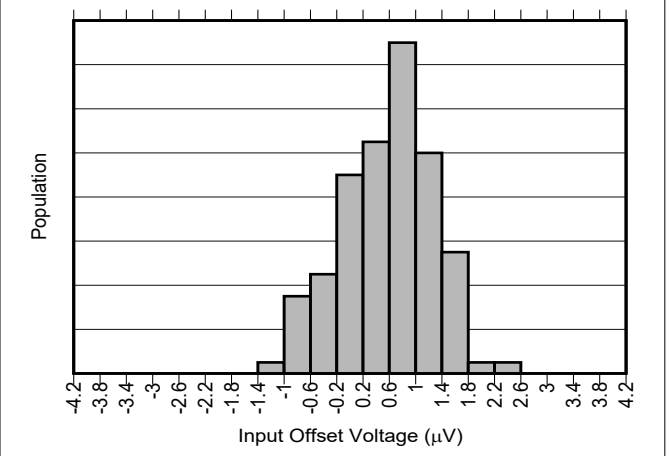
图 7-4. INA296A5 输入失调电压产生分布图
