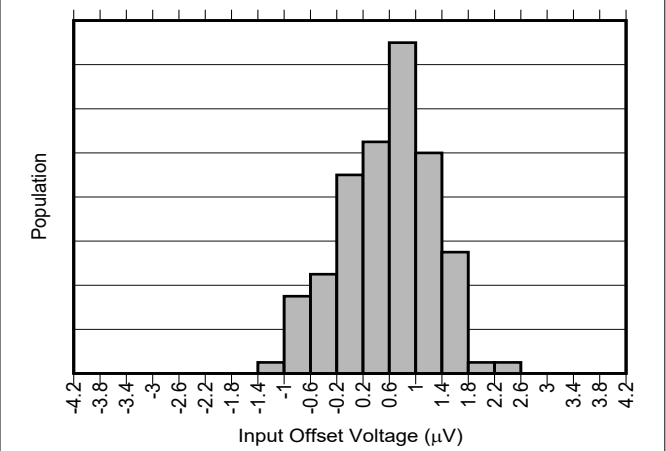
图 7-4. INA296A5 输入失调电压产生分布图
