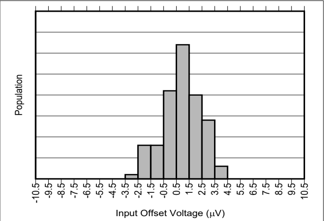
图 7-2. INA296A2 输入失调电压产生分布图
