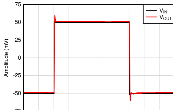
图 6-56. 大信号稳定时间 (下降沿)
