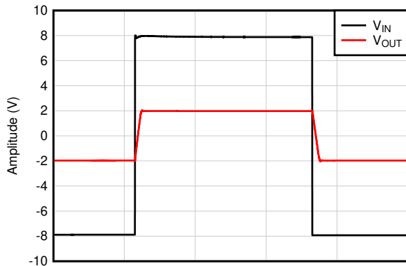
图 6-53. 大信号稳定时间 (下降沿)
