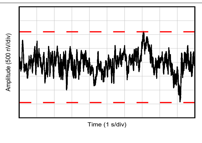
图 5-12. 0.1Hz 至 10Hz 噪声
