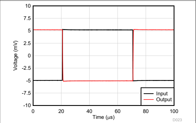
图 5-28. 过载恢复
