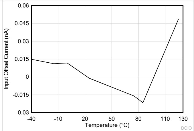
图 6-10. 输入失调电流与温度间的关系
