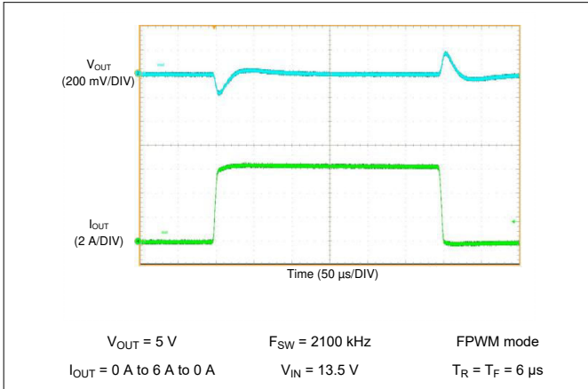
图 9-53. LM61460 Load Transient
