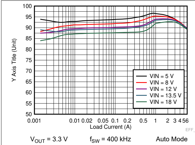
图 9-3. LM73606-Q1 Efficiency
