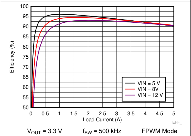
图 9-6. LM73605-Q1 Efficiency
