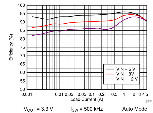
图 9-5. LM73605-Q1 Efficiency
