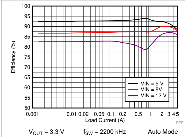
图 9-7. LM73605-Q1 Efficiency
