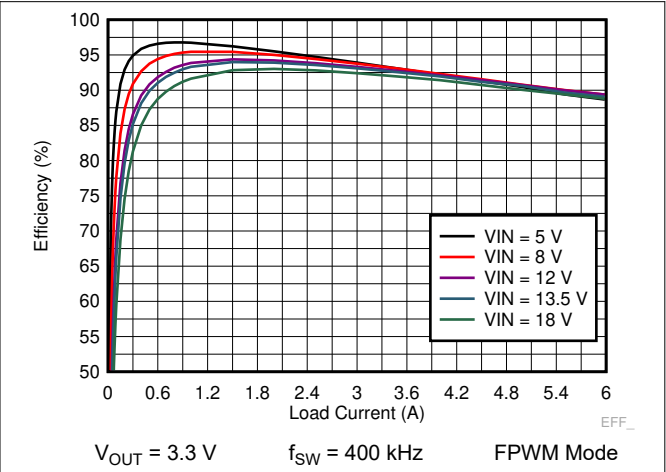
图 9-4. LM73606-Q1 Efficiency
