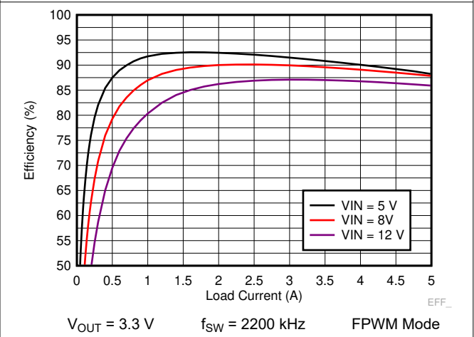
图 9-8. LM73605-Q1 Efficiency
