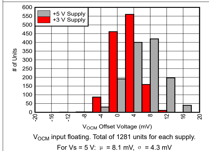
图 7-23. Common-Mode Output Offset from V_{s+} / 2 Default Value
