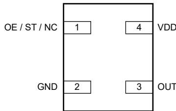
图 5-2. LMK6C 4-Pin VSON (Top View)
