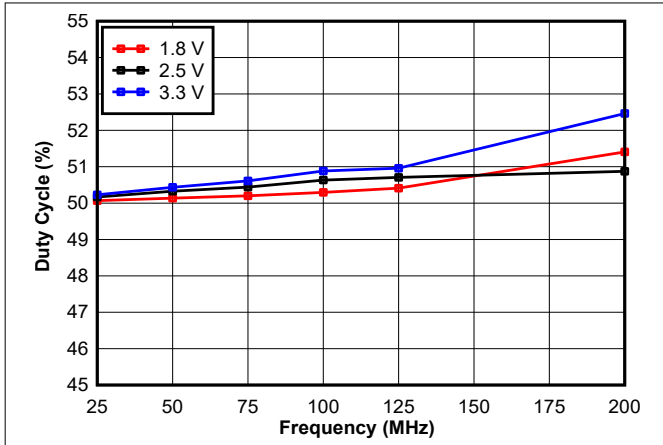
图 6-25. 占空比 (%) 与频率和电源电压间的关系；25°C
