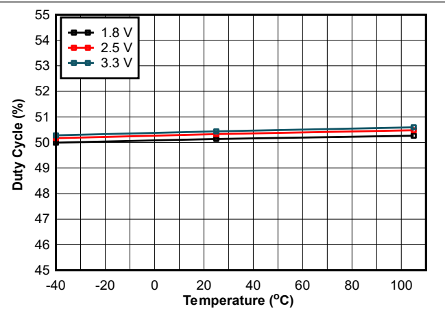
图 6-26. 占空比 (%) 与温度和电源间的关系；频率 50MHz
