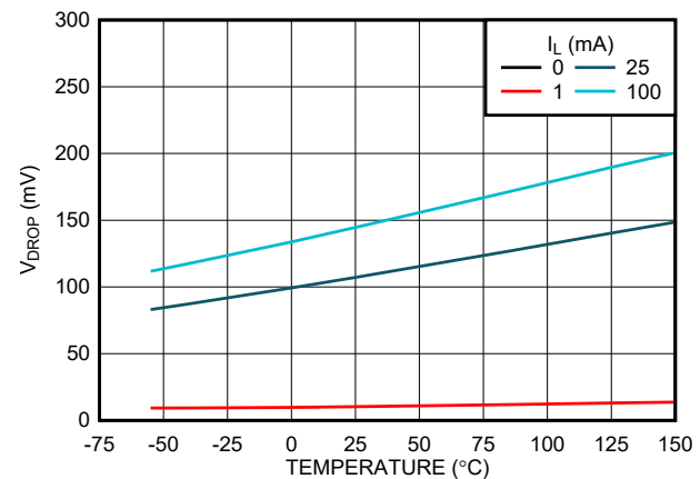
压降电压与温度间的关系 (新芯片)
