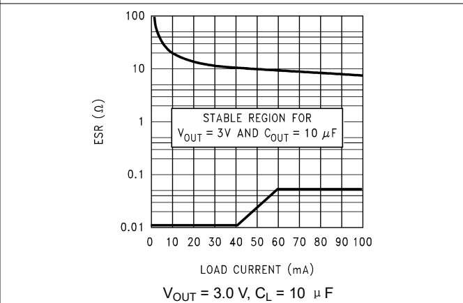
图 7-6. 3.0-V, 10- \mu\text{F} ESR Curves (Legacy Chip)
