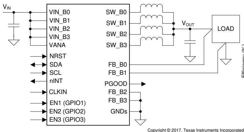
简化原理图
