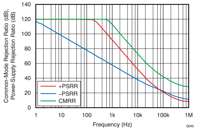
图 10. CMRR 和 PSRR 与频率间的关系 (以输入为基准)
