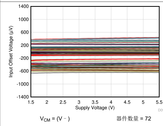
图 6-12. 偏移电压与电源电压间的关系
