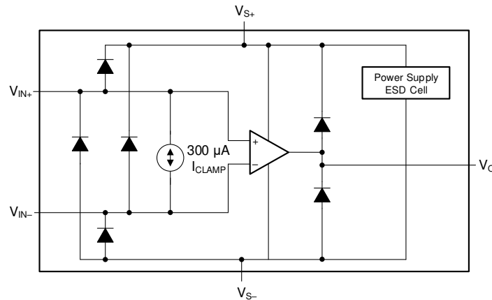
图 7-2. Internal ESD Protection
