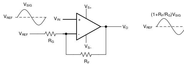
图 8-1. Noninverting Amplifier
