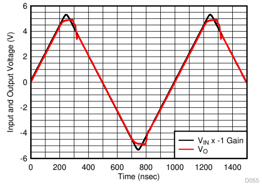
图 6-14. Output Overdrive Recovery
