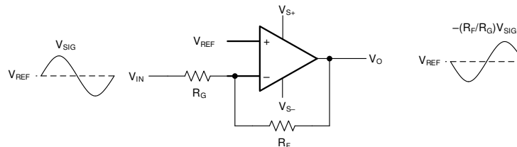
图 8-2. Inverting Amplifier
