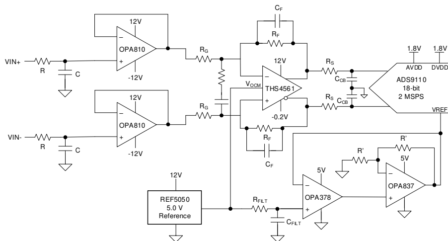
高阻抗输入数据采集前端
