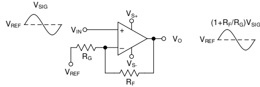
图 8-3. Noninverting Amplifier
