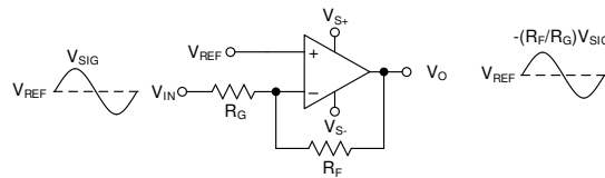
图 8-4. Inverting Amplifier
