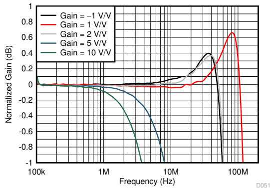
See 图 8-1 and 图 8-2, V_O = 20\text{ mV}_{PP}
