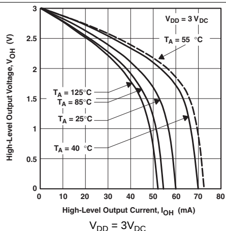
图 5. 高电平输出电压与高电平输出电流间的关系
