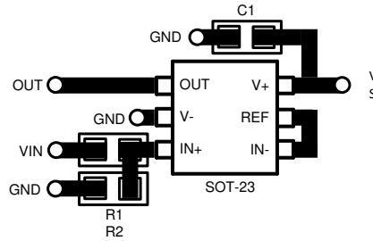
图 10-7. 布局示例
