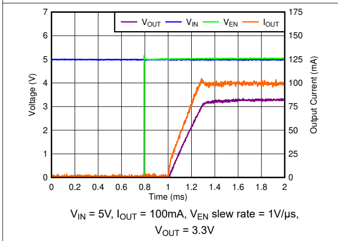
图 5-11. EN Start-Up
