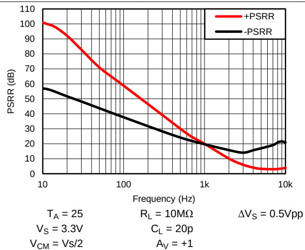
Figure 24. \pm\text{PSRR} 与频率间的关系
