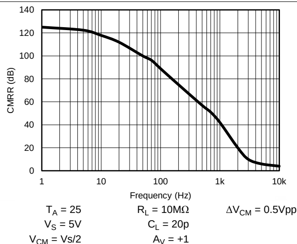
Figure 23. CMRR 与频率间的关系
