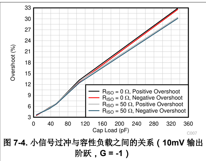
图 7-3. 小信号过冲与容性负载之间的关系 ( 10\text{mV} 输出阶跃, G = 1 )
