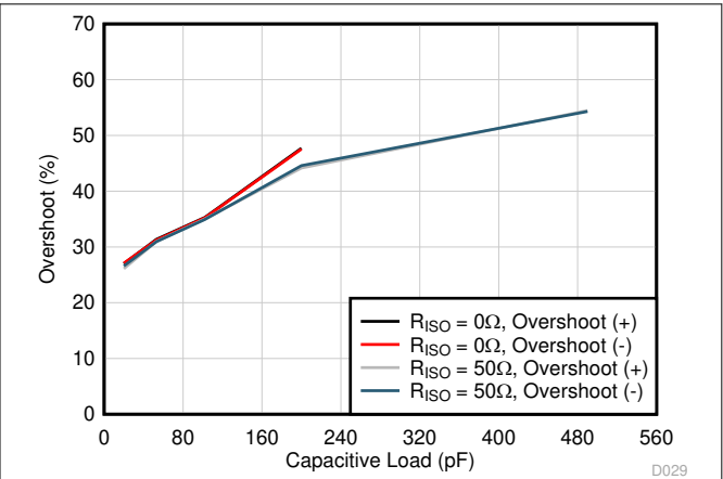
图 7-4. 小信号过冲与容性负载之间的关系 (20mV pp 输出阶跃, G = -1)
