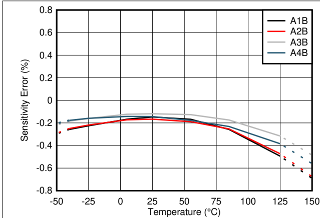
图 7-1. TMCS1101AxB 灵敏度误差与温度间的关系
