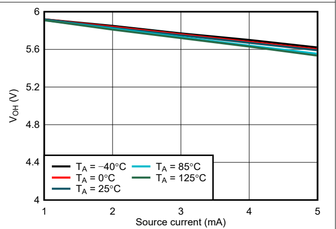
图 7-17. WDO V_{OH} 与 I_{source} 间的关系, V_{DD} = 6.0\text{V}
