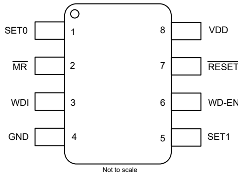
图 6-3. 引脚配置选项 C DDF 封装，8 引脚 SOT-23， TPS35-Q1 顶视图
