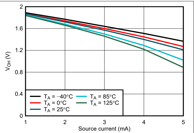
图 7-15. WDO V_{OH} 与 I_{source} 间的关系, V_{DD} = 2.0\text{V}
