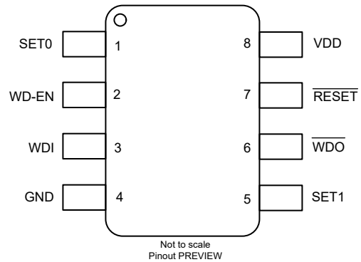
图 6-4. 引脚配置选项 D DDF 封装，8 引脚 SOT-23， TPS35-Q1 顶视图
