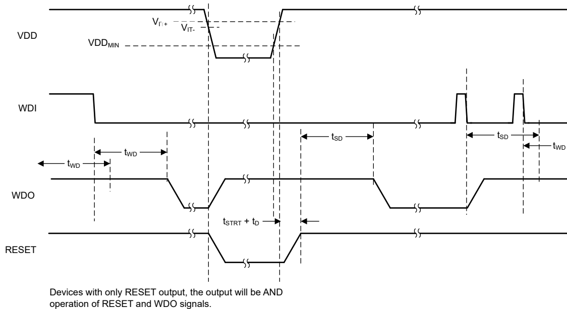
图 8-13. 输出锁存器时序行为
