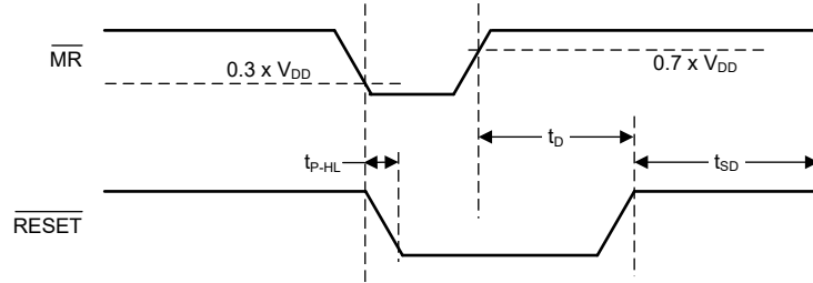
图 8-12. \overline{MR} 引脚响应
