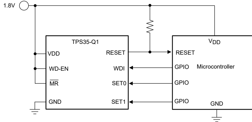
图 9-1. 微控制器电源和看门狗监控电路
