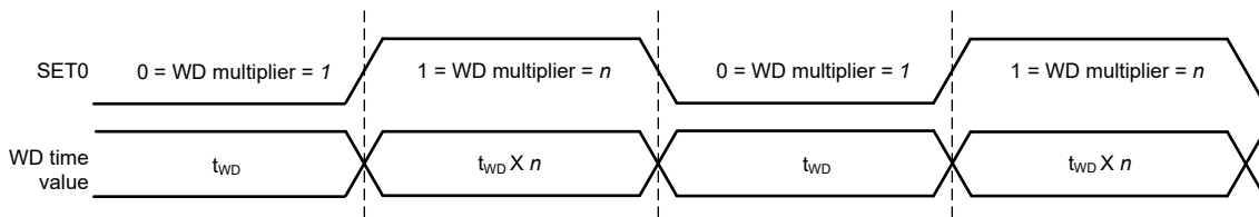
图 8-10. 具有 2 个 SET 引脚的看门狗运行情况
