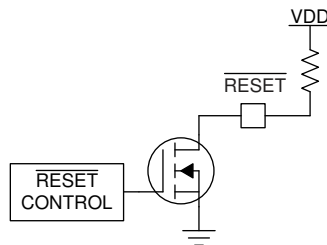
图 9-2. 开漏 \overline{\text{RESET}} 配置
