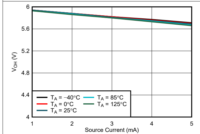
图 7-16. RESET V_{OH} 与 I_{source} 间的关系, V_{DD} = 6.0\text{V}
