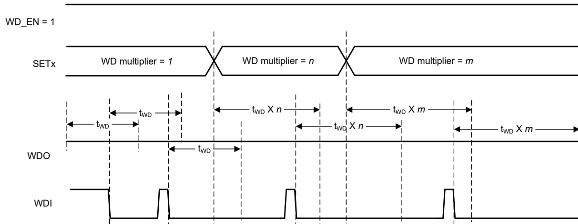
图 8-9. 具有 SETx 引脚状态的看门狗行为
