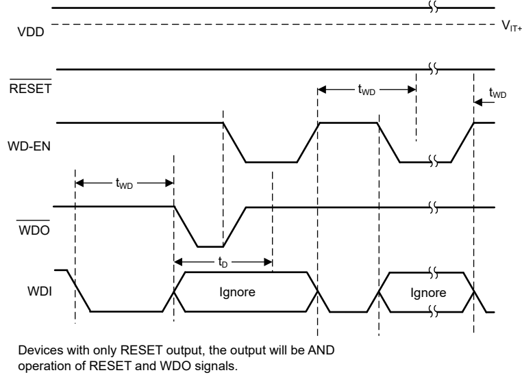
图 8-7. 看门狗启用：WD-EN 引脚控制
