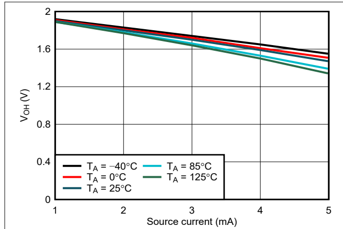
图 7-14. RESET V_{OH} 与 I_{source} 间的关系, V_{DD} = 2.0\text{V}
