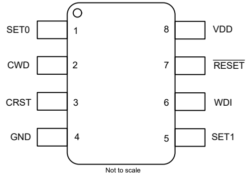
图 6-2. 引脚配置选项 B DDF 封装，8 引脚 SOT-23， TPS35-Q1 顶视图
