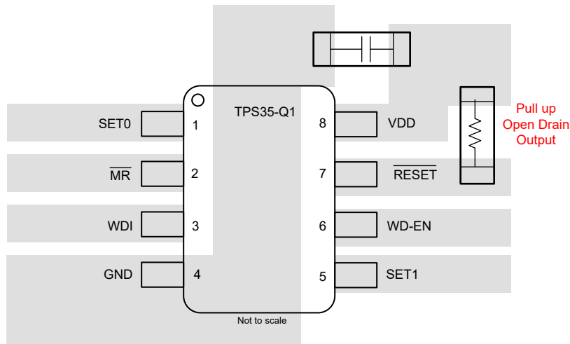
图 11-1. 引脚排列 C 的典型布局 - TPS35-Q1
