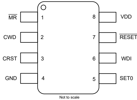
图 6-1. 引脚配置选项 A DDF 封装，8 引脚 SOT-23， TPS35-Q1 顶视图
