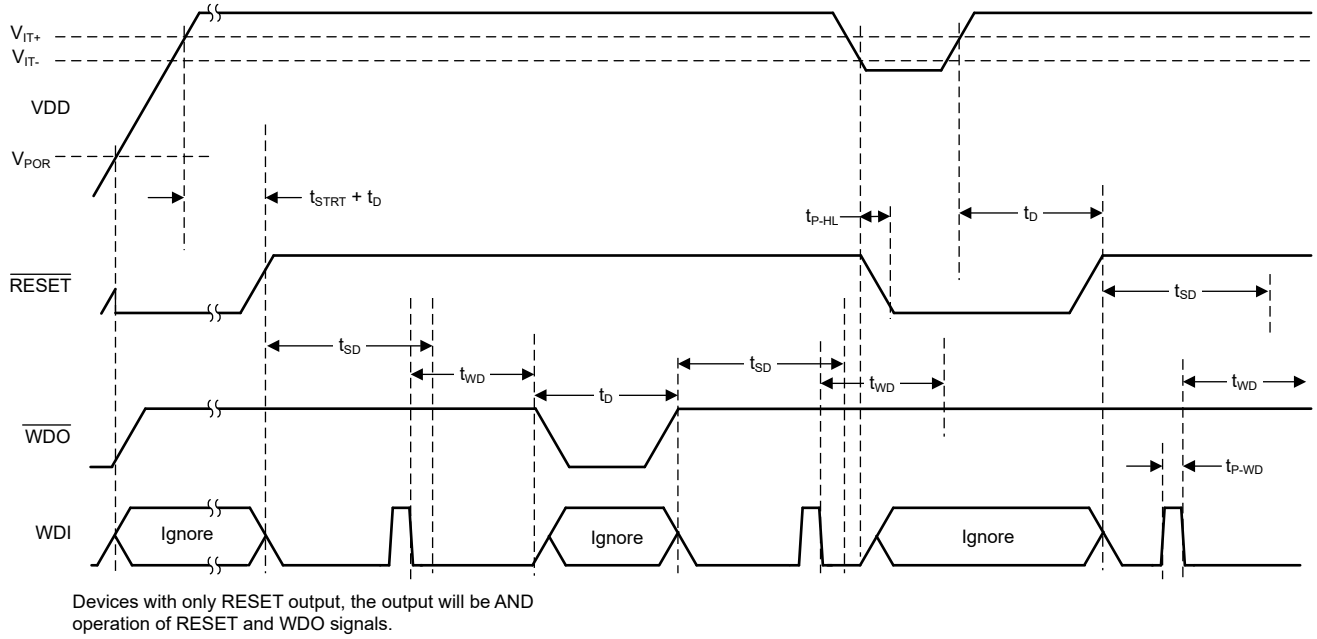
图 7-1. 功能时序图
