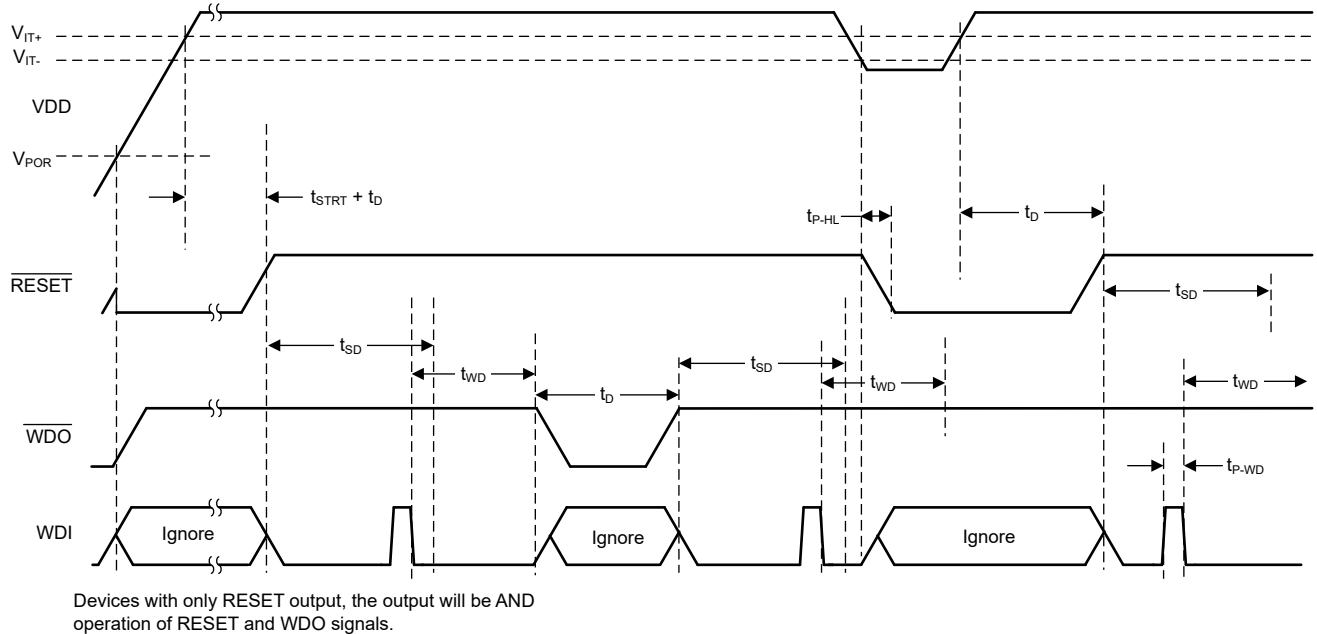
图 8-5. 电压监控器时序图
