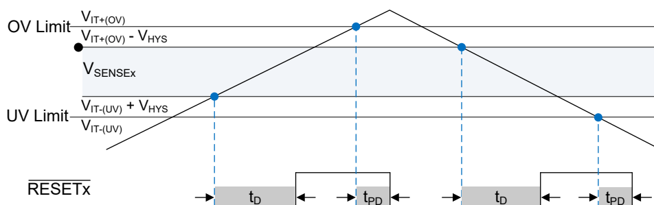
图 7-6. RESETx Output
