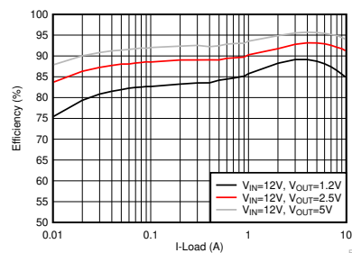
效率与输出电流，500kHz，Eco-mode
