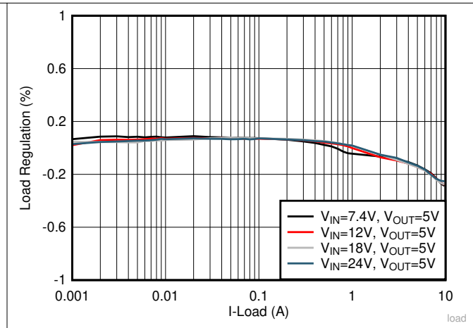
图 8-3. Load Regulation
