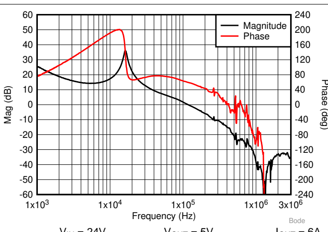
图 21. Bode Plot
