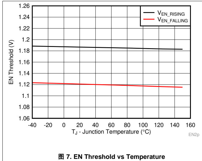
图 7. EN Threshold vs Temperature
