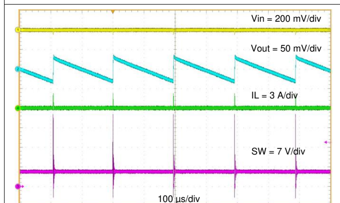
图 20. Line Regulation
