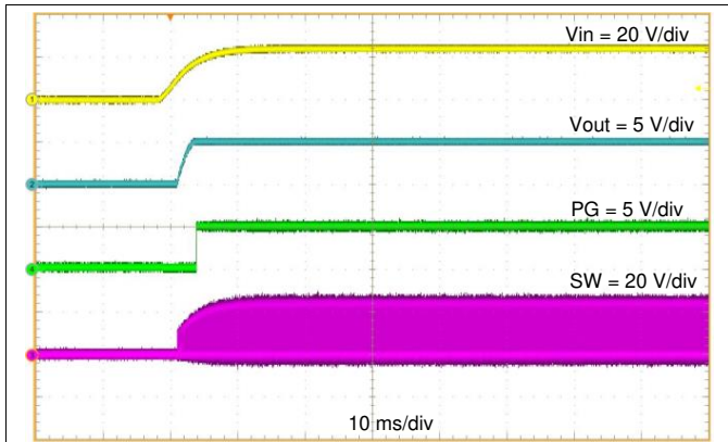
图 30. Startup Relative to V_{IN}
