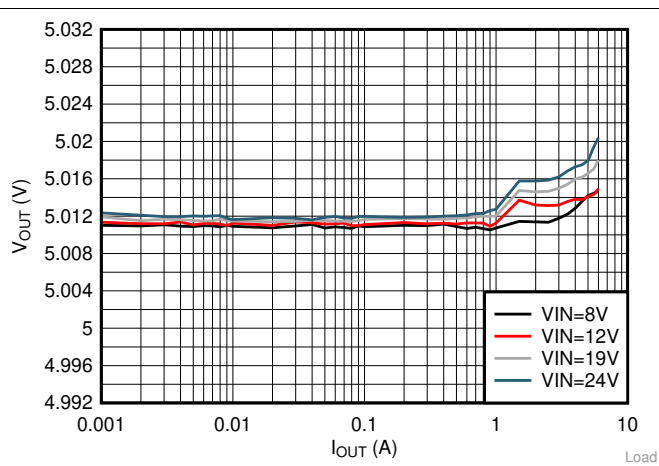
图 19. Load Regulation
