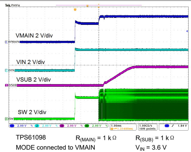
图 9-37. Startup
