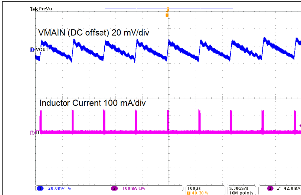
图 9-3. Switching Waveforms
