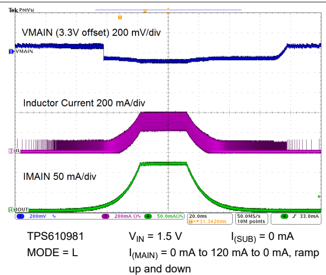
图 9-18. Load Regulation
