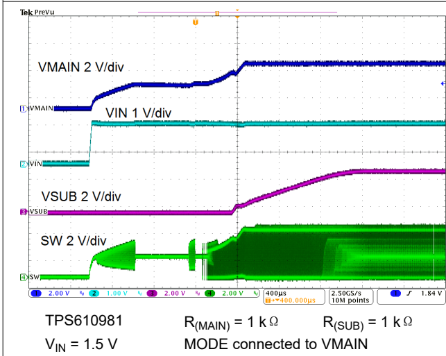
图 9-23. Startup
