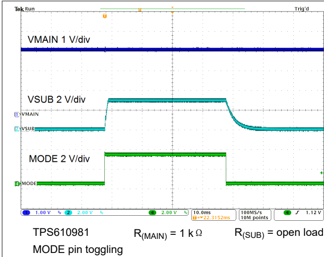
图 9-21. Mode Toggling
