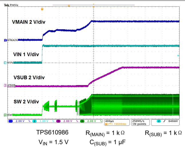
图 9-22. Startup
