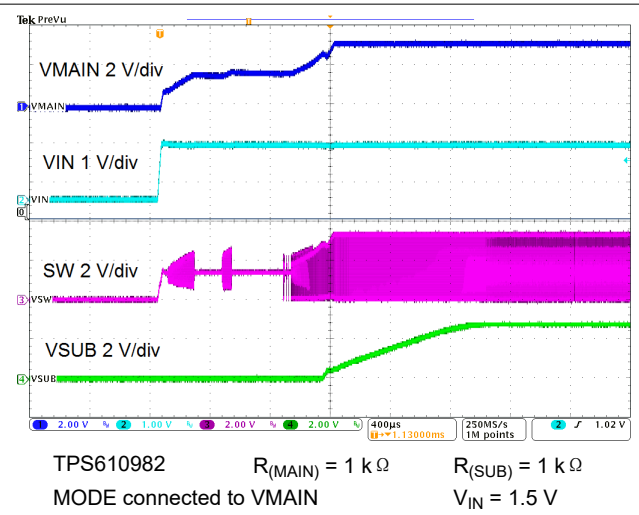
图 9-39. Startup
