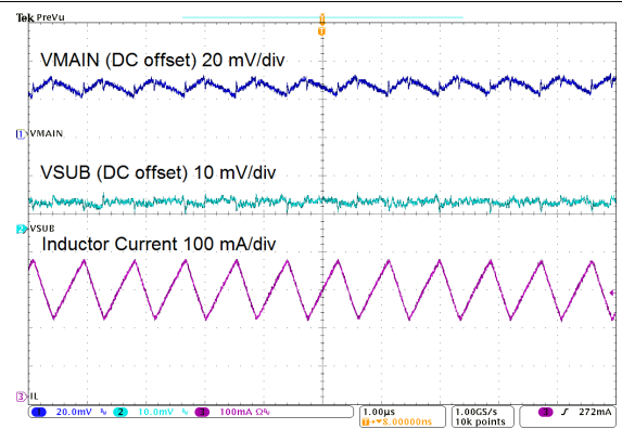
图 9-6. Switching Waveforms
