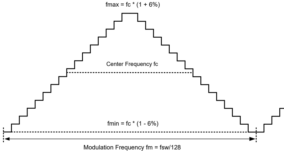
图 9-7. 展频频谱图
