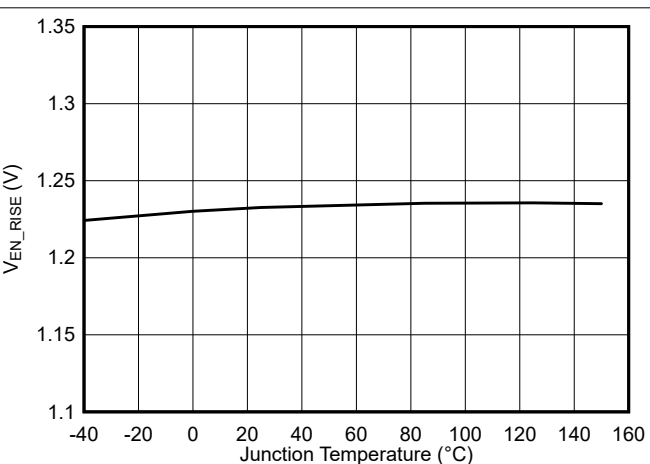
图 8-6. 启用阈值与结温间的关系
