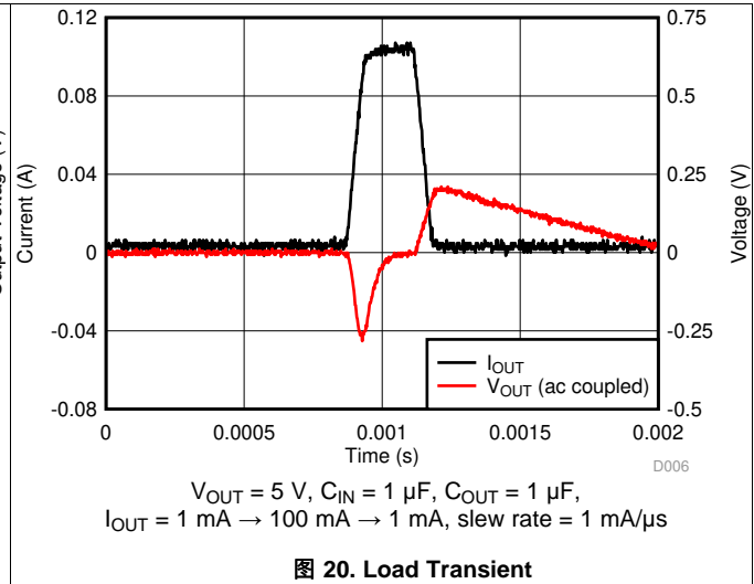
图 20. Load Transient
