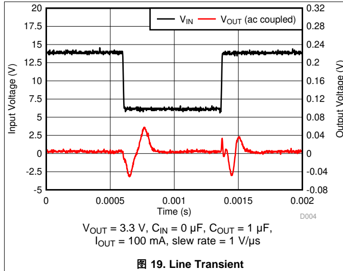
图 19. Line Transient
