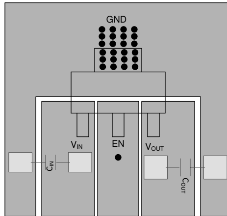
图 10-1. SOT-223 (DCY) Layout
