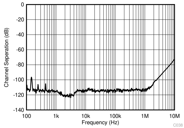
图 7-30. 通道隔离与频率间的关系
