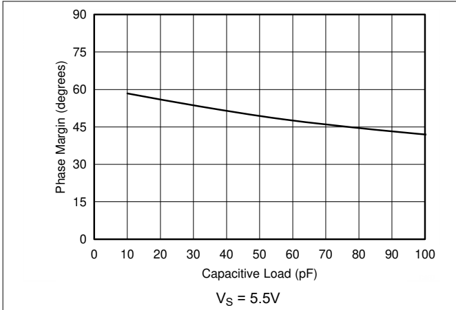
图 7-31. 相位裕度与容性负载间的关系
