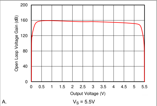
图 7-32. 开环电压增益与输出电压间的关系
