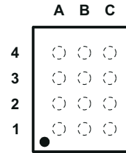
图 5-2. NMN 封装 , 12 引脚 nFPGA ( 顶视图 )
