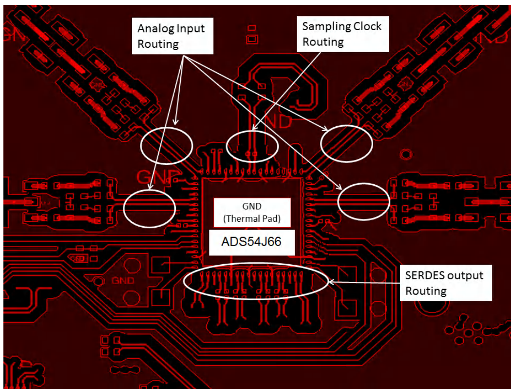
图 8-10. ADS54J66EVM Layout
