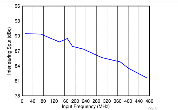
图 6-20. IL Spur vs Input Frequency
