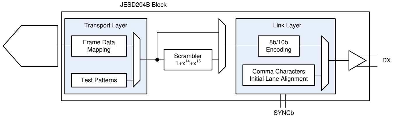
图 7-25. JESD Interface Block Diagram
