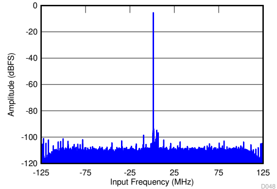
图 6-50. FFT for 370-MHz Input Signal
